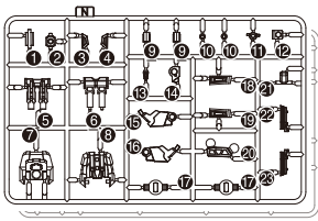
Nパーツ (×2)
